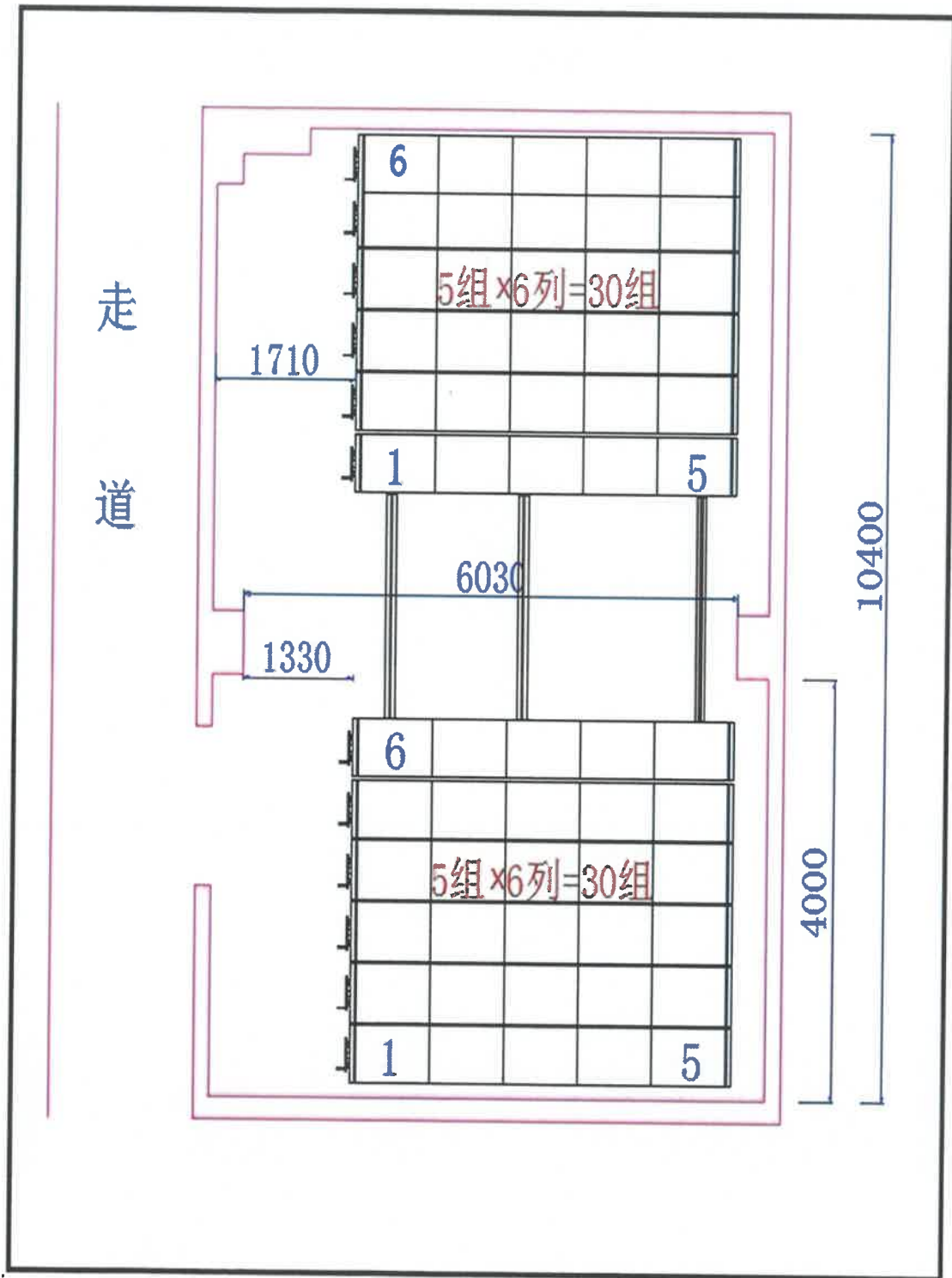
密集文件柜室内分布图
